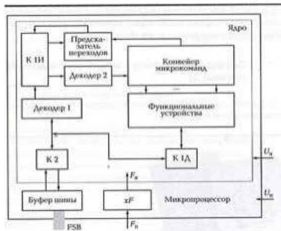
Рисунок 2 Упрощенная структурная схема процессора
