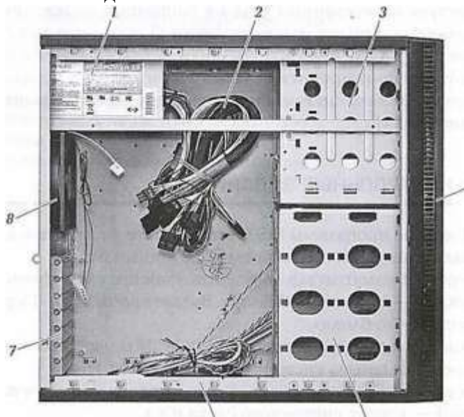
Рисунок 5. Вид корпуса системного блока со стороны монтажа
