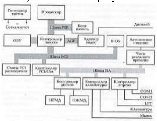
Рисунок 1 Структурная схема ПЭВМ
